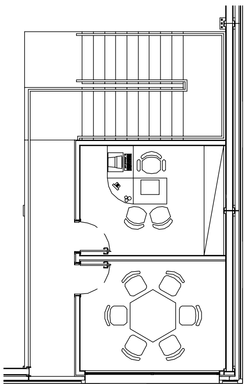
planta piso 1 escala . 1/100
